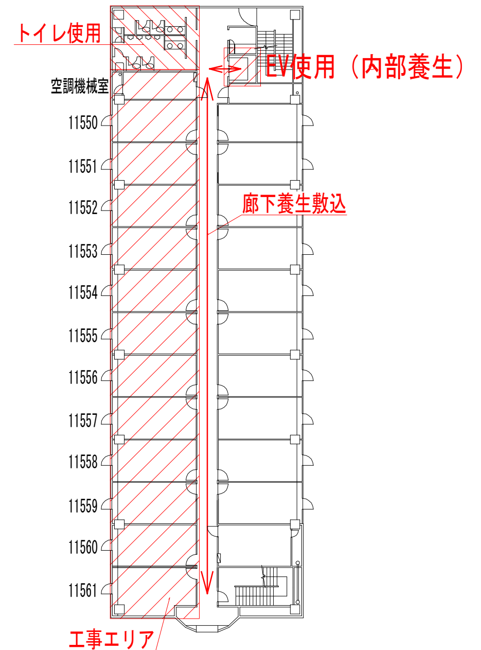
B棟5階平面図
